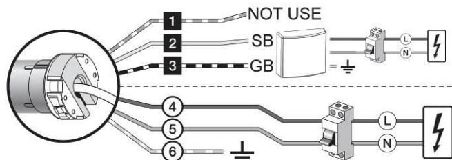
Schema connessione di un motore Radio integrato Nice con TTBUS
